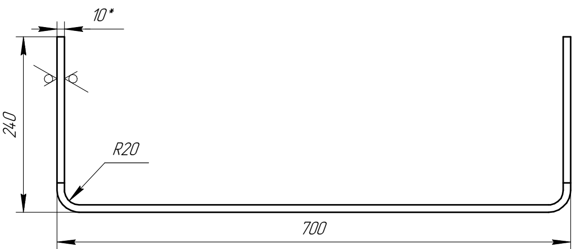
Дет. поз. 1
