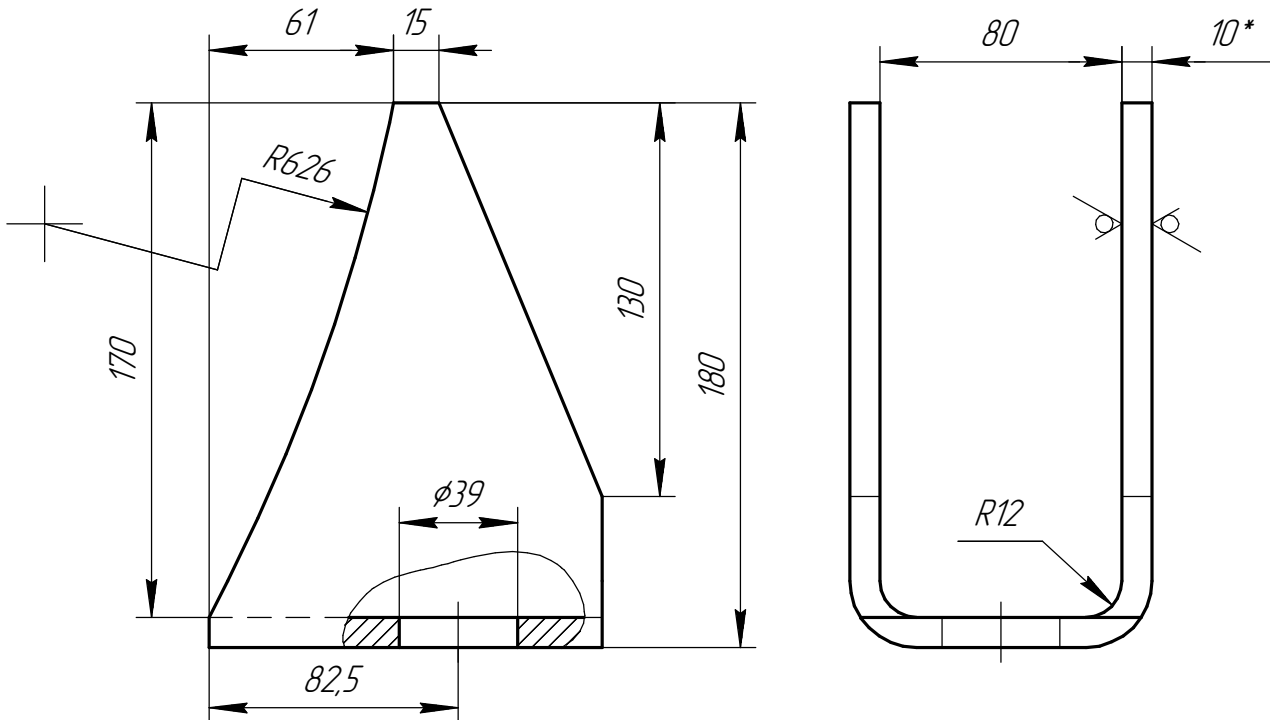
Дет. поз. 5 (1:2,5)
